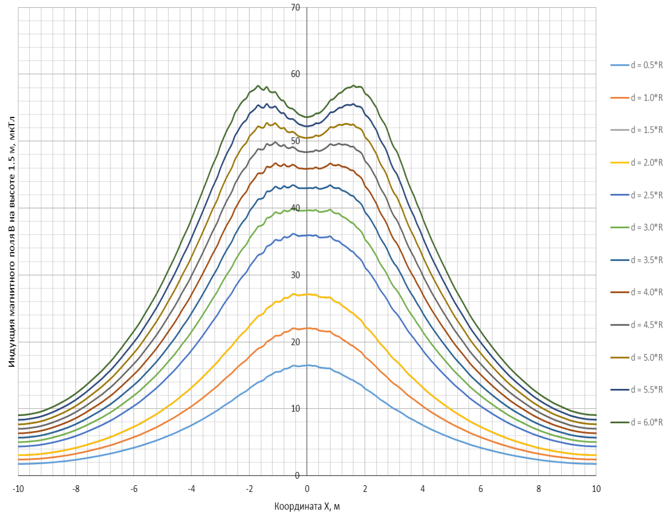
Магнитное поле В двух подземных кабельных линий на высоте 1.5 м над поверхностью земли
