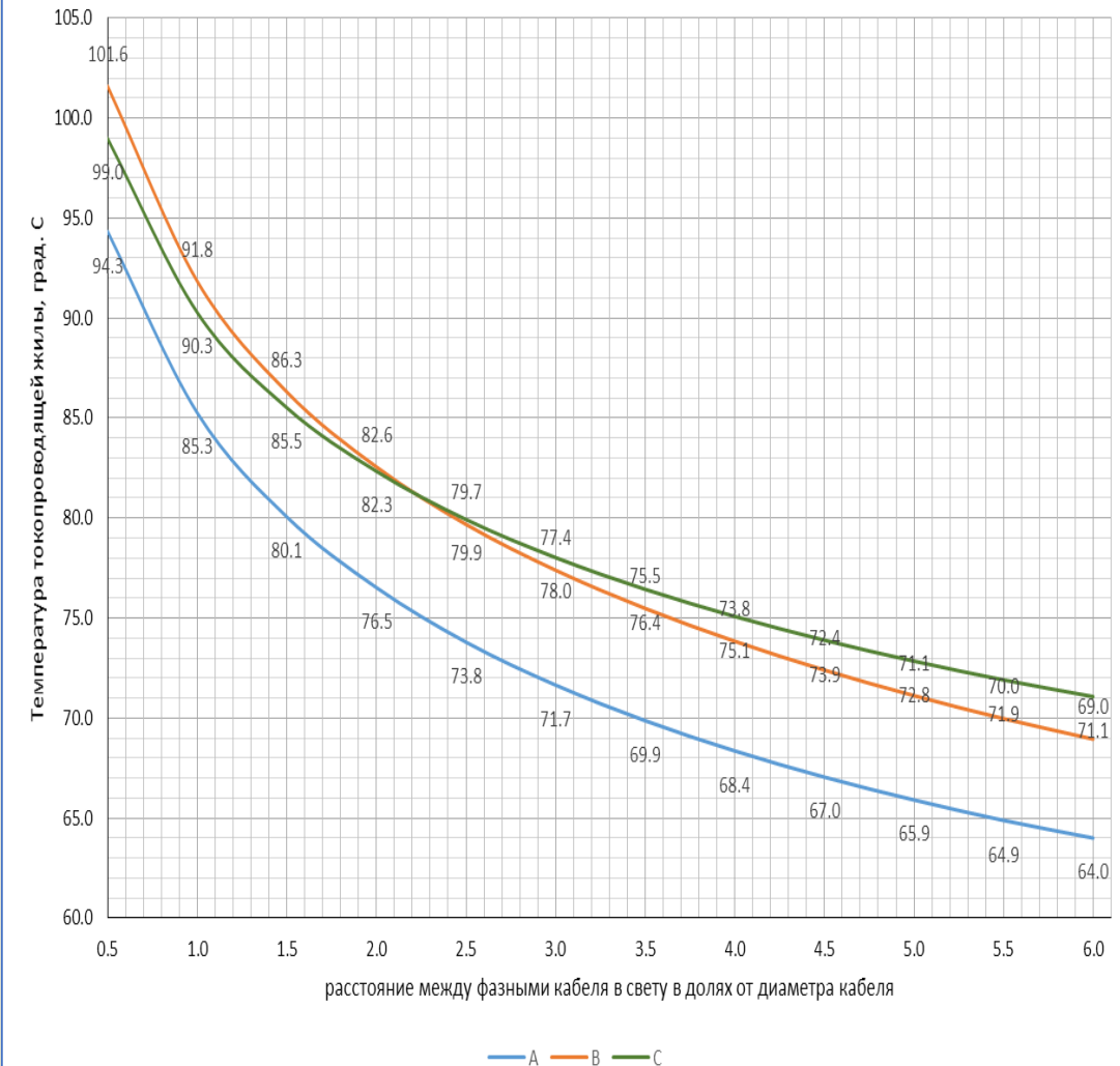
Температуры фазных жил в зависимости от расстояния между фазами
