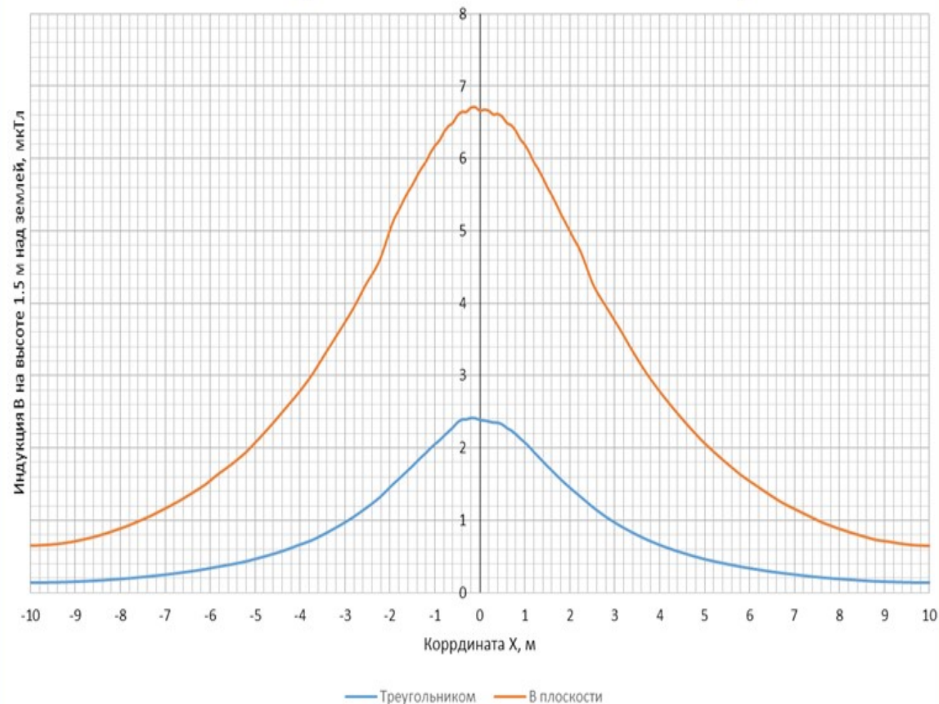
Магнитное поле одиночной кабельной линии без магнитного экрана
