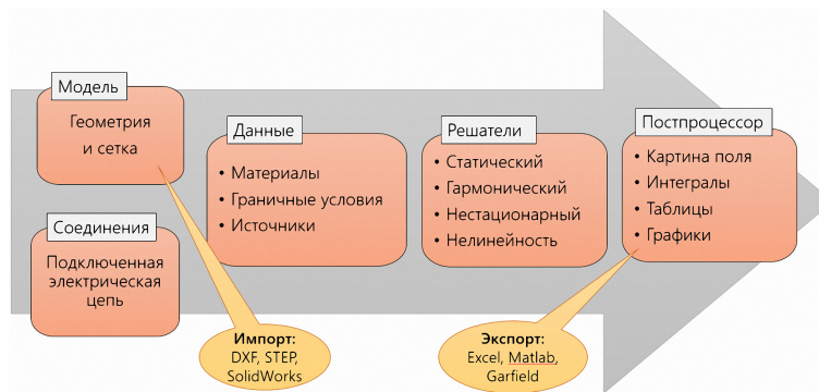
Рис. 4. – Подсистемы программы ELCUT
