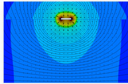
Рис. 6. – Соотношение между волновой и квазистатической формулировками
