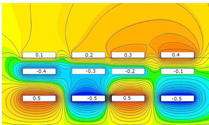
Рис. 10. – Электрическое поле системы нескольких проводников
