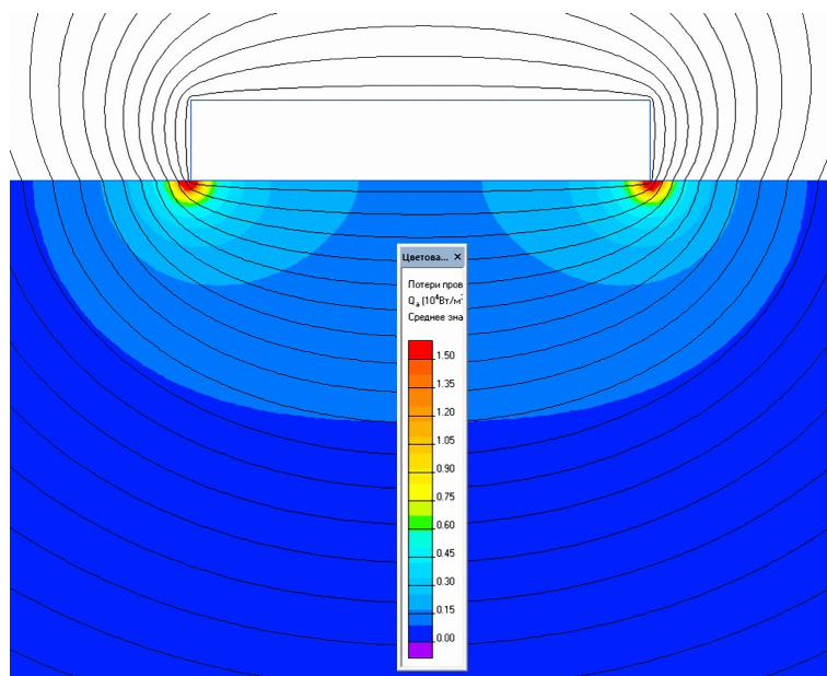
Рис. 7. – Электрическое поле с учетом потерь в диэлектрике
