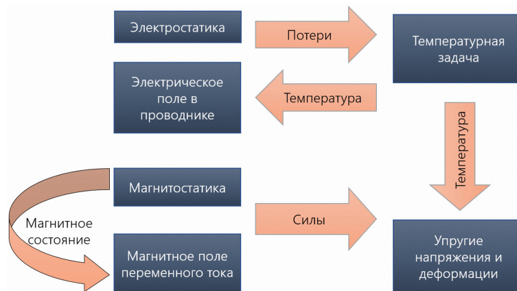
Рис. 3. – Мультифизические связи между отдельными постановками задач
