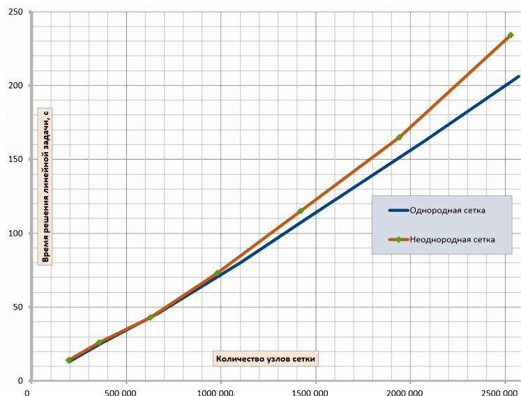
Рис. 5. – Зависимость времени решения от размерности задачи
